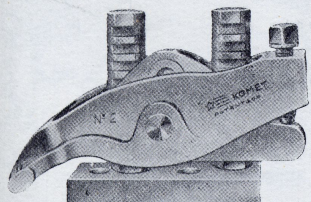
Brida de sujeción regulable n.º 2
