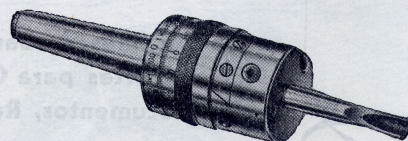
Cabezales de mandrilado micrométrico
